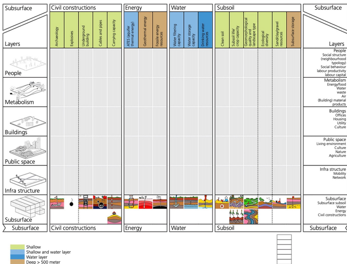
Figura 1 | System Exploration Environment and Subsurface (SEES), con la “superficie” sull'asse Y e il “sottosuolo” sull'asse X, utilizzato per integrare le condizioni del sottosuolo nello sviluppo urbano. Fonte: Hooimeijer e Maring, 2013.
